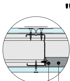
پیچ LN سازه پشتیبان SP60
